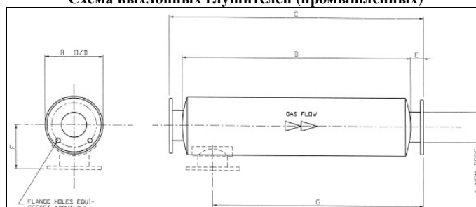
Схема выхлопных глушителей (промышленных)
