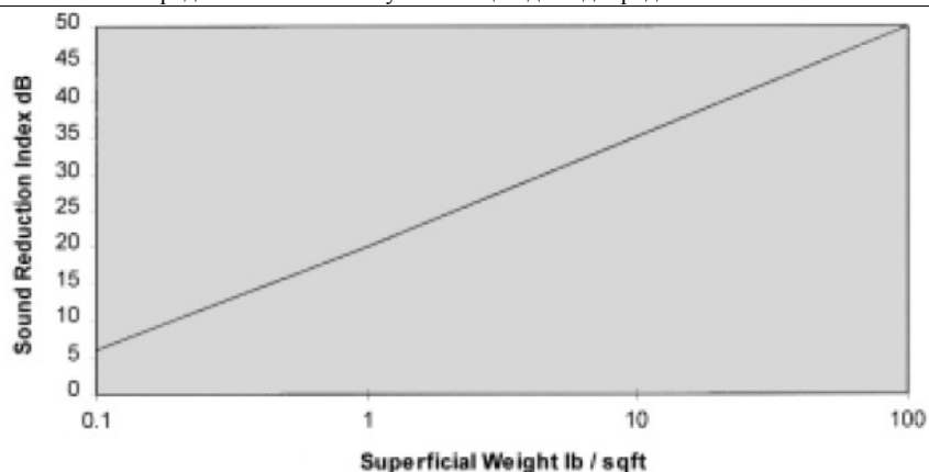
Средние показатели звукоизоляции для однородных панелей
