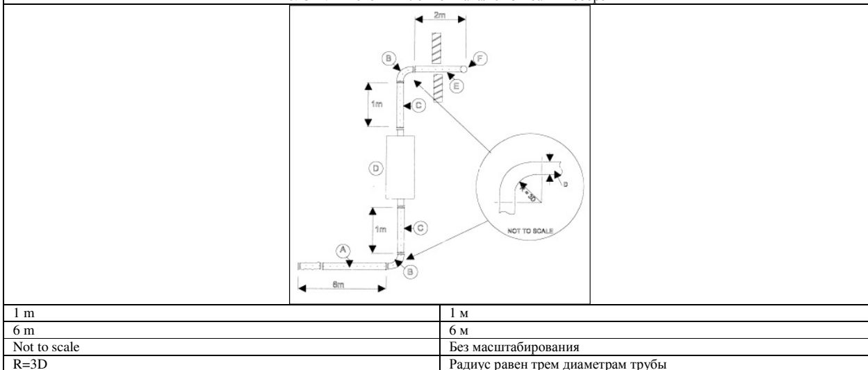
Рис. C12. Номограмма глушителя и прямых участков
