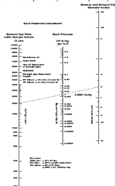
Рис. C12. Номограмма глушителя и прямых участков
