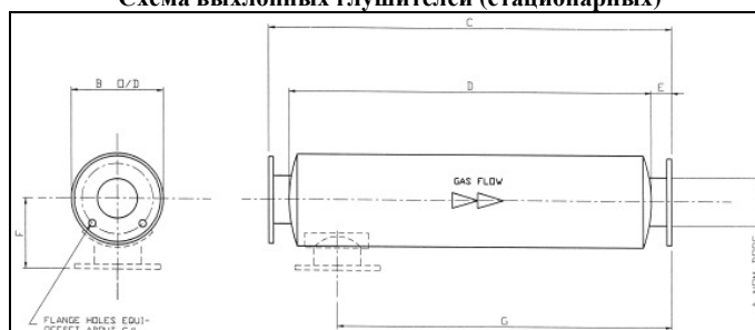
Схема выхлопных глушителей (стационарных)
