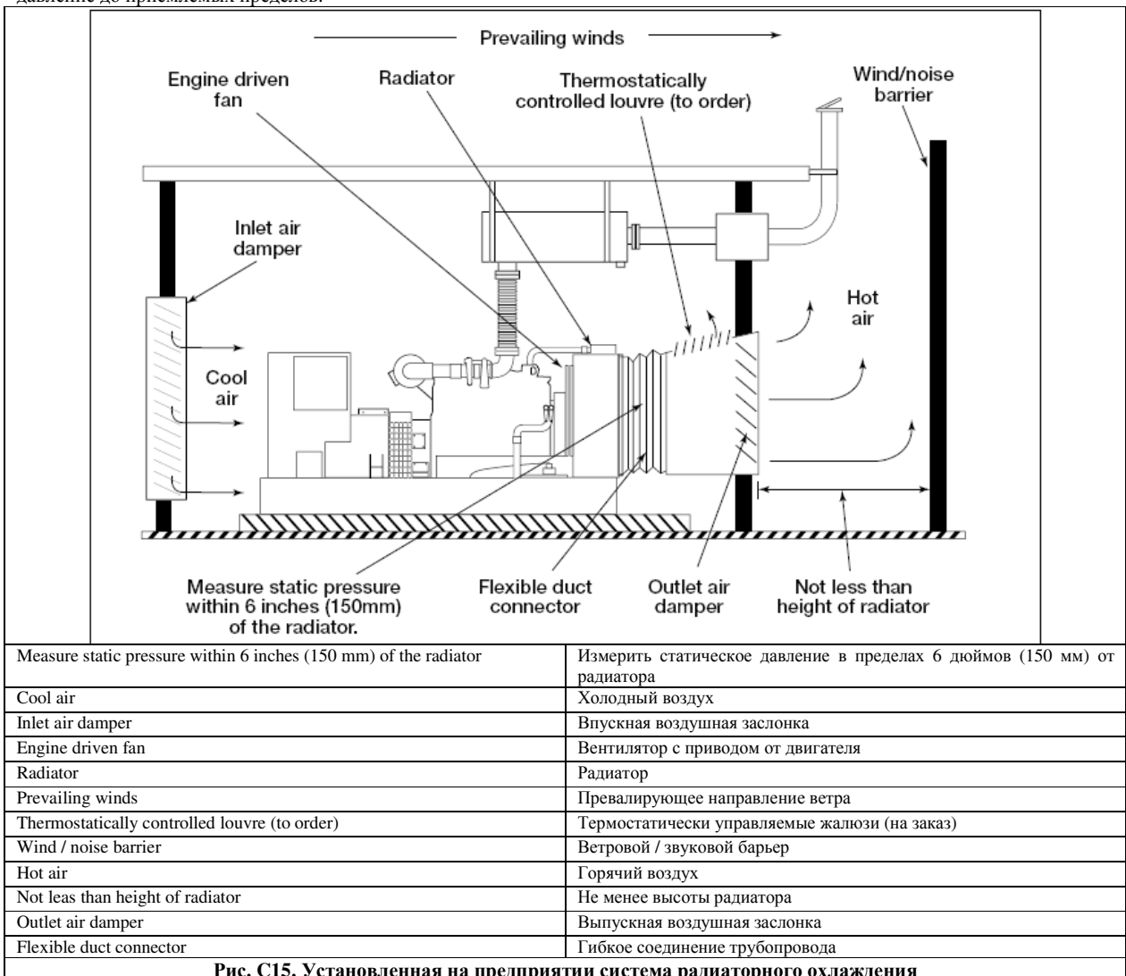
Рис. C15. Установленная на предприятии система радиаторного охлаждения
