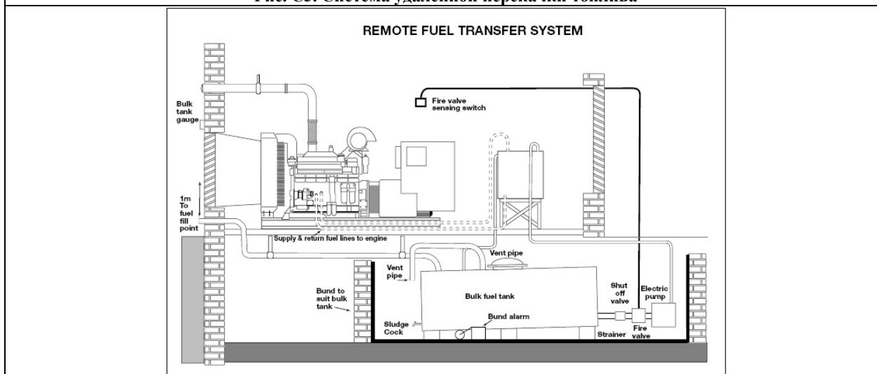
Рис. С5. Система удаленной перекачки топлива
