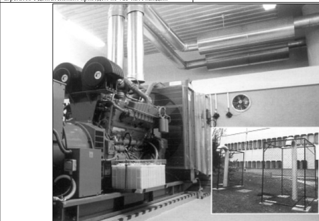
Двойной выхлопной канал с теплоизоляцией и оболочкой из алюминиевой фольги от 12-цилиндрового агрегата Cummins 640 кВА / 50 Гц с двумя двигателями VTA28 с турбонаддувом
