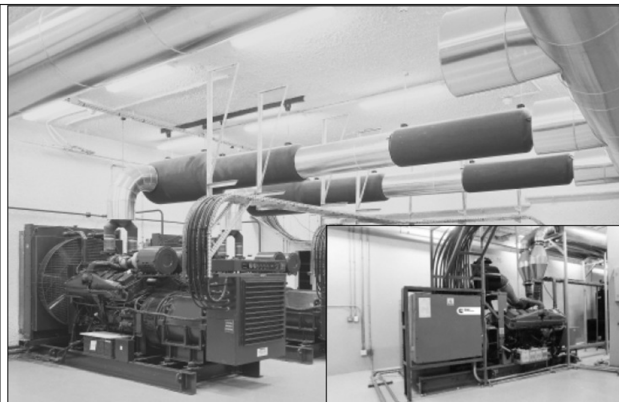
Хороший пример чистого и хорошо изолированного выхлопного канала от двух 12-цилиндровых дежурных агрегатов с двигательным приводом по 725 кВА каждый
