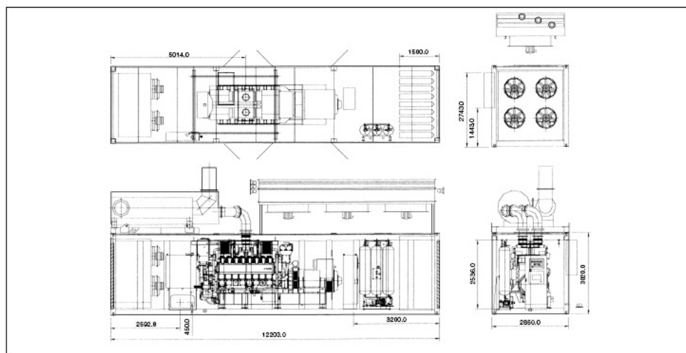
Модель GQMBna 1570 кВт с двигателем 16-цилиндровым V-образным двигателем QSV81G
