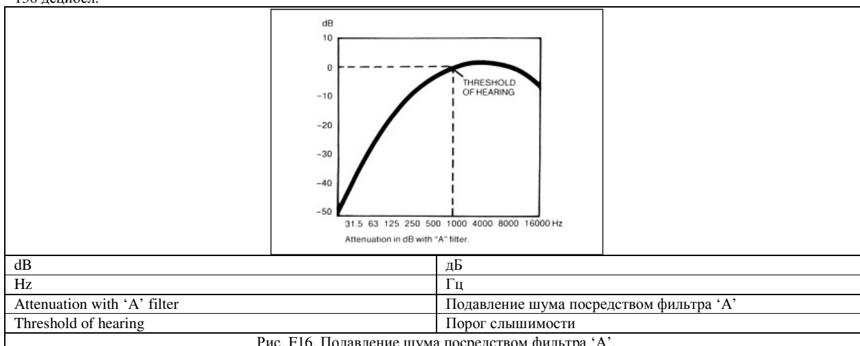
Рис. F16. Подавление шума посредством фильтра 'A'.
