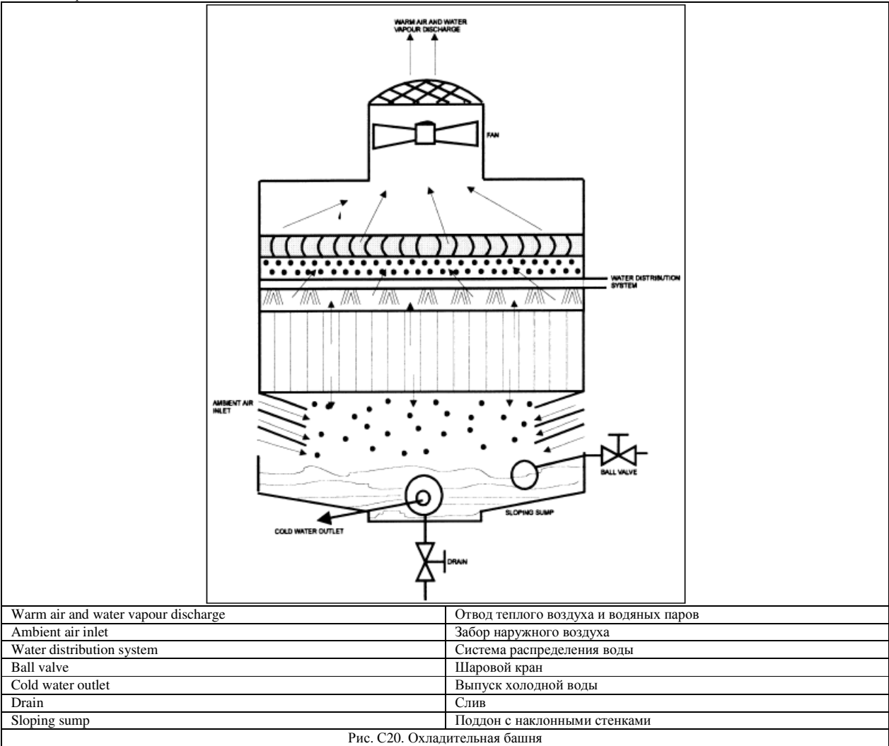
Рис. C20. Охладительная башня
