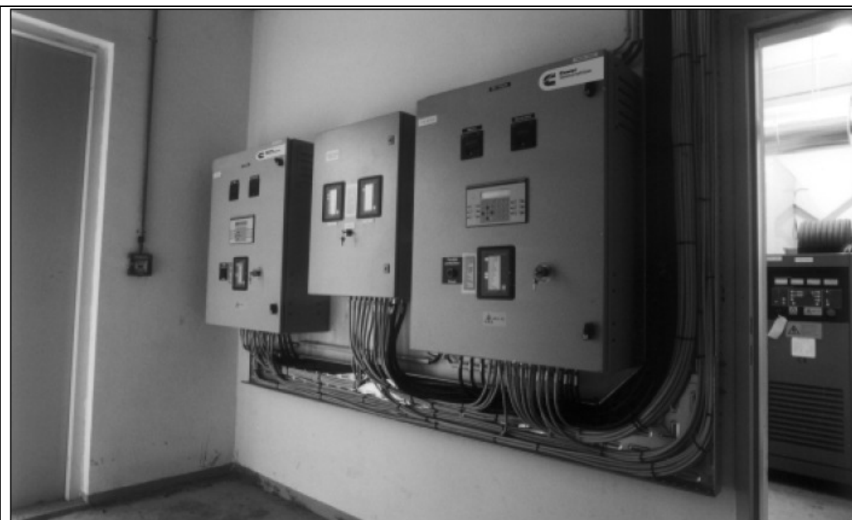
Главные контроллеры MC150 в составе автоматической системы параллельного подключения
