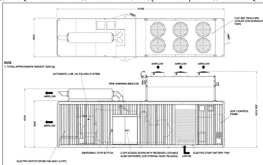
Модель GQMBna 1750 кВт с двигателем 18-цилиндровым V-образным двигателем QSV91G
