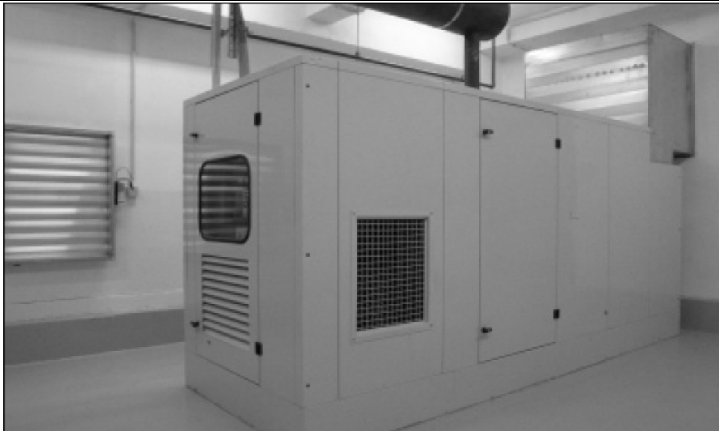
Сверхмалощумный генераторный агрегат Cummins на 110 кВА, установленный в акустически обработанном машинном зале. Метод позволяет достичь сверхнизких уровней звука в местах, чувствительных к шуму, таких как этот отель «Хилтон».
